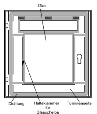
Abb. 2 – Türinnenseite mit eingebauter Dichtung
